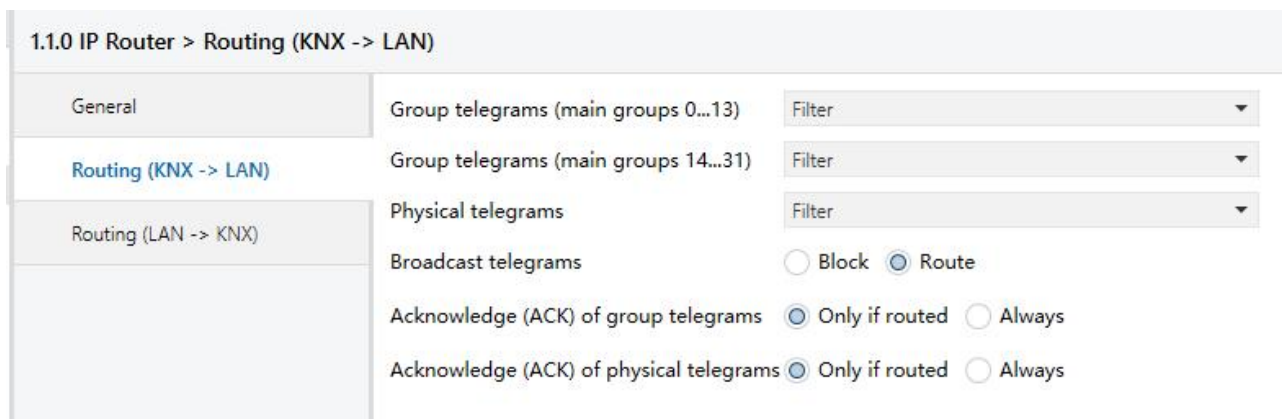
图 5.2 “Routing(KNX->LAN)”参数设置界面
