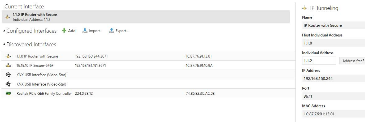
图 5.6.1 ETS 总线接口配置界面
