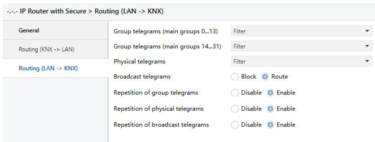
图 5.3 “Routing(LAN->KNX)”参数设置界面
