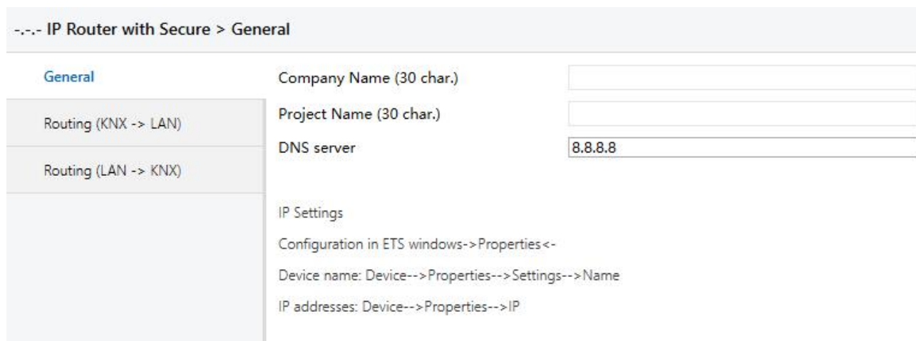
图 5.1 "General"参数设置界面
