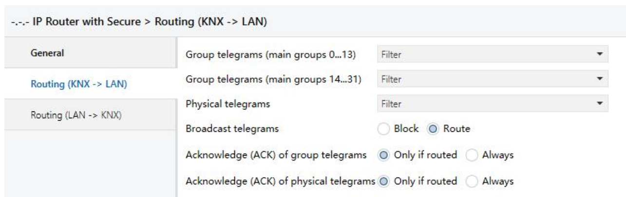
图 5.2 “Routing(KNX->LAN)”参数设置界面
